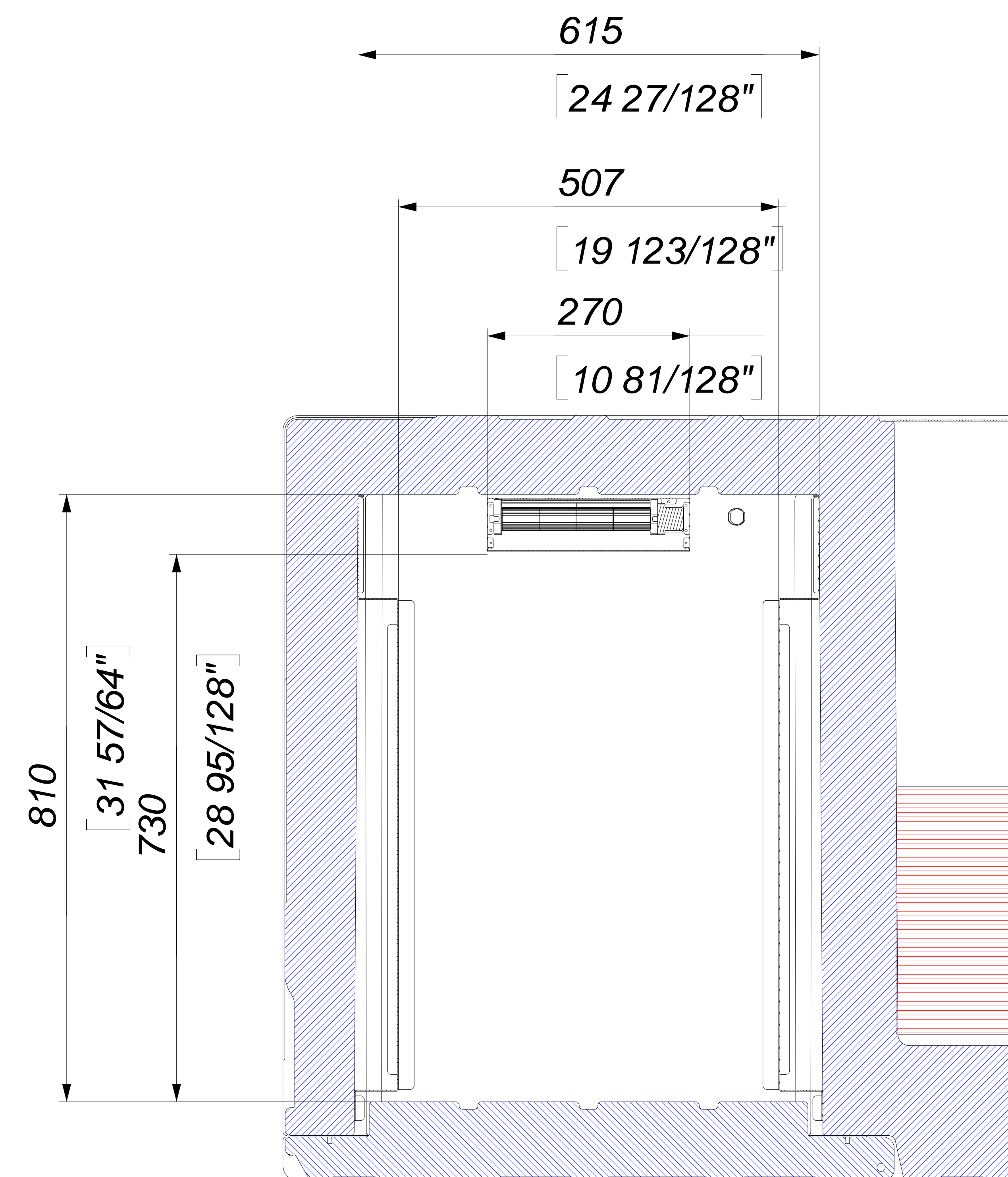
Sezione F-F SCALE 1 : 4
