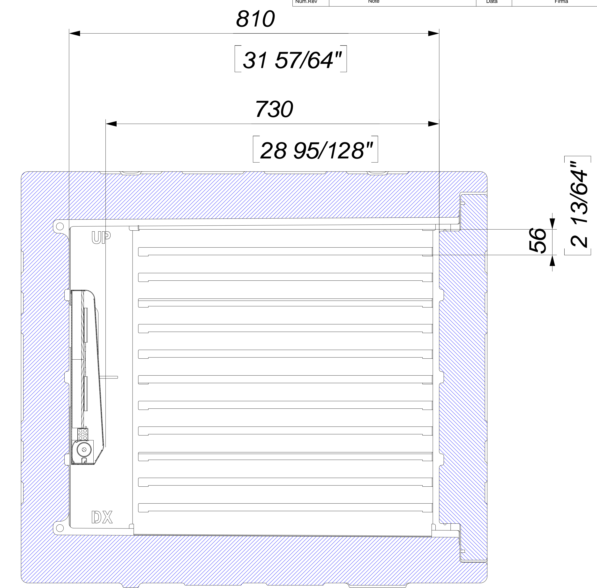
Sezione E-E SCALE 1 : 4
