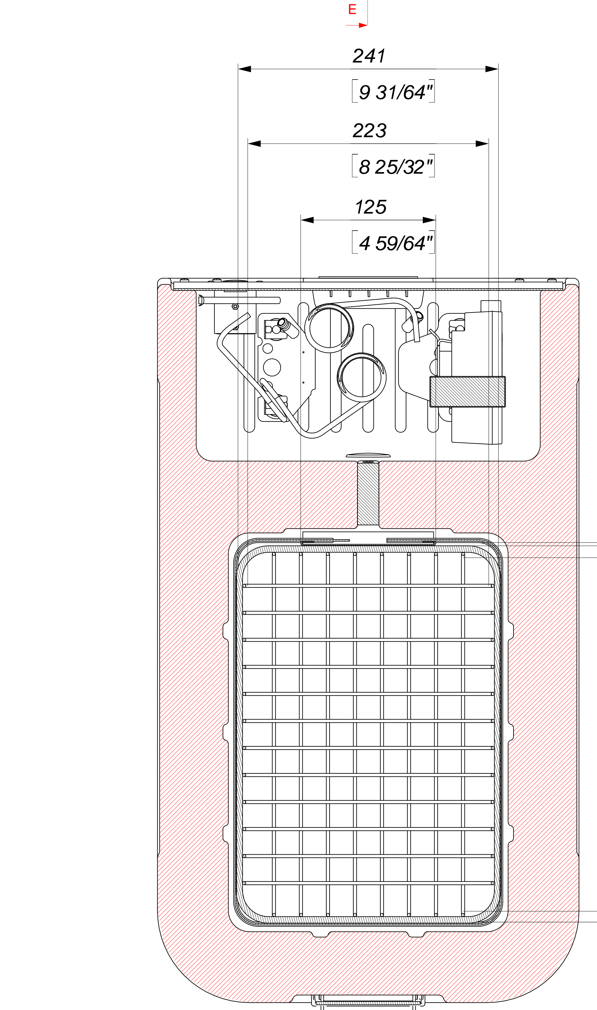
Sezione F-F SCALE 1:2
