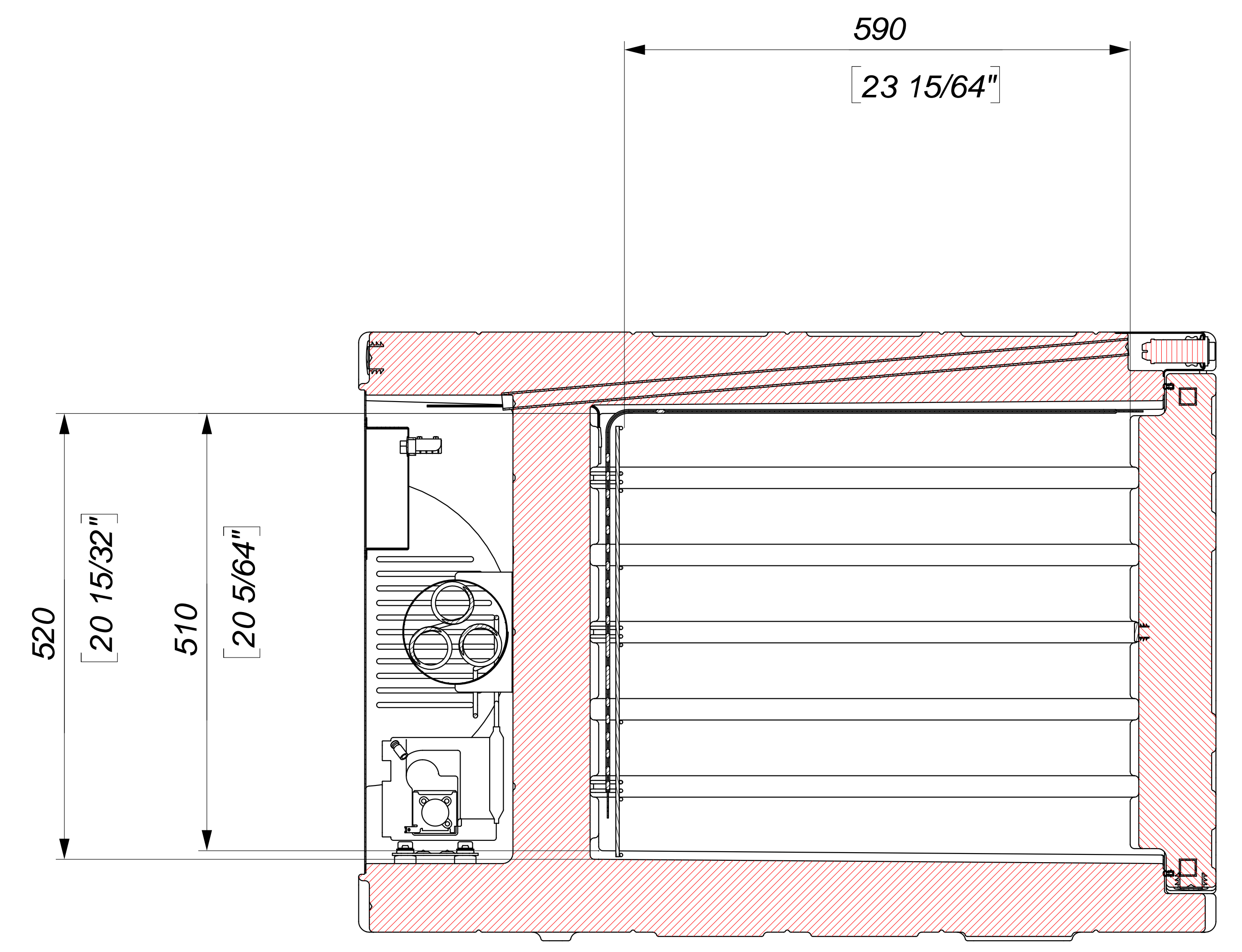
Sezione E-E SCALE 1 : 4
