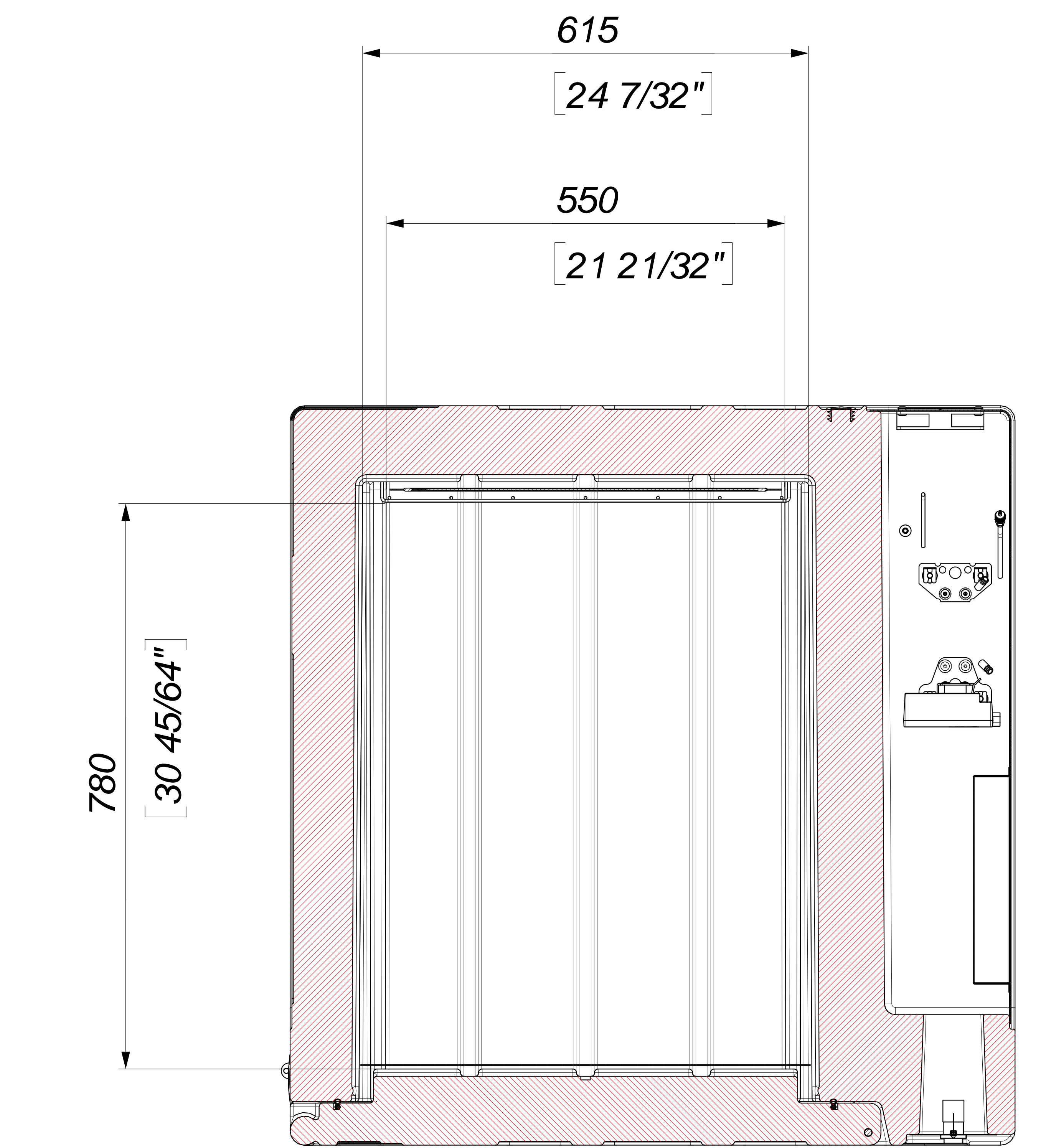
Sezione F-F SCALE 1 : 4
