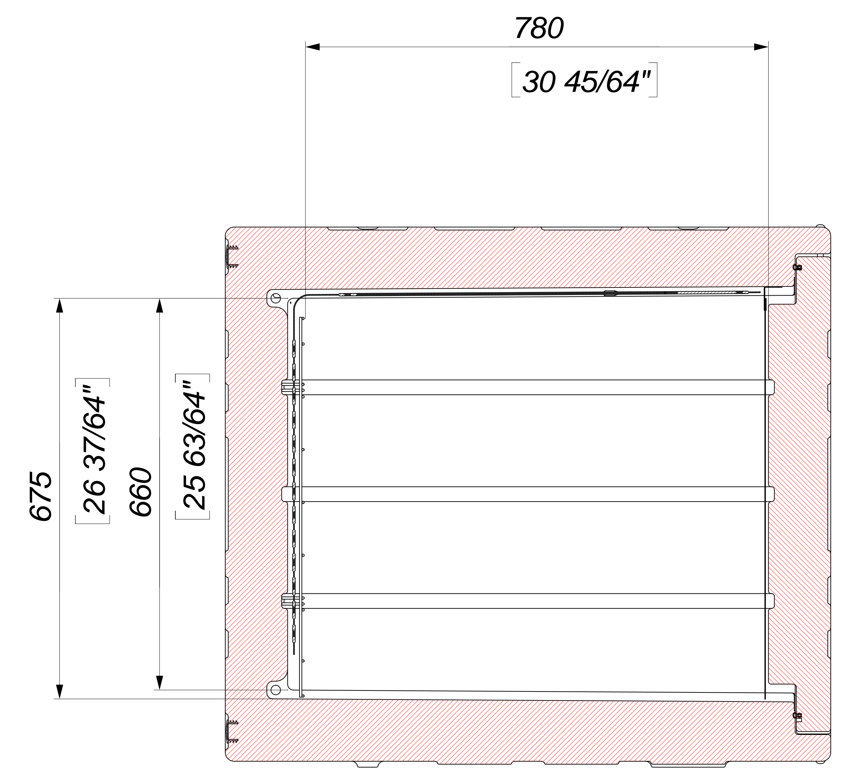
Sezione E-E SCALE 1 : 4
