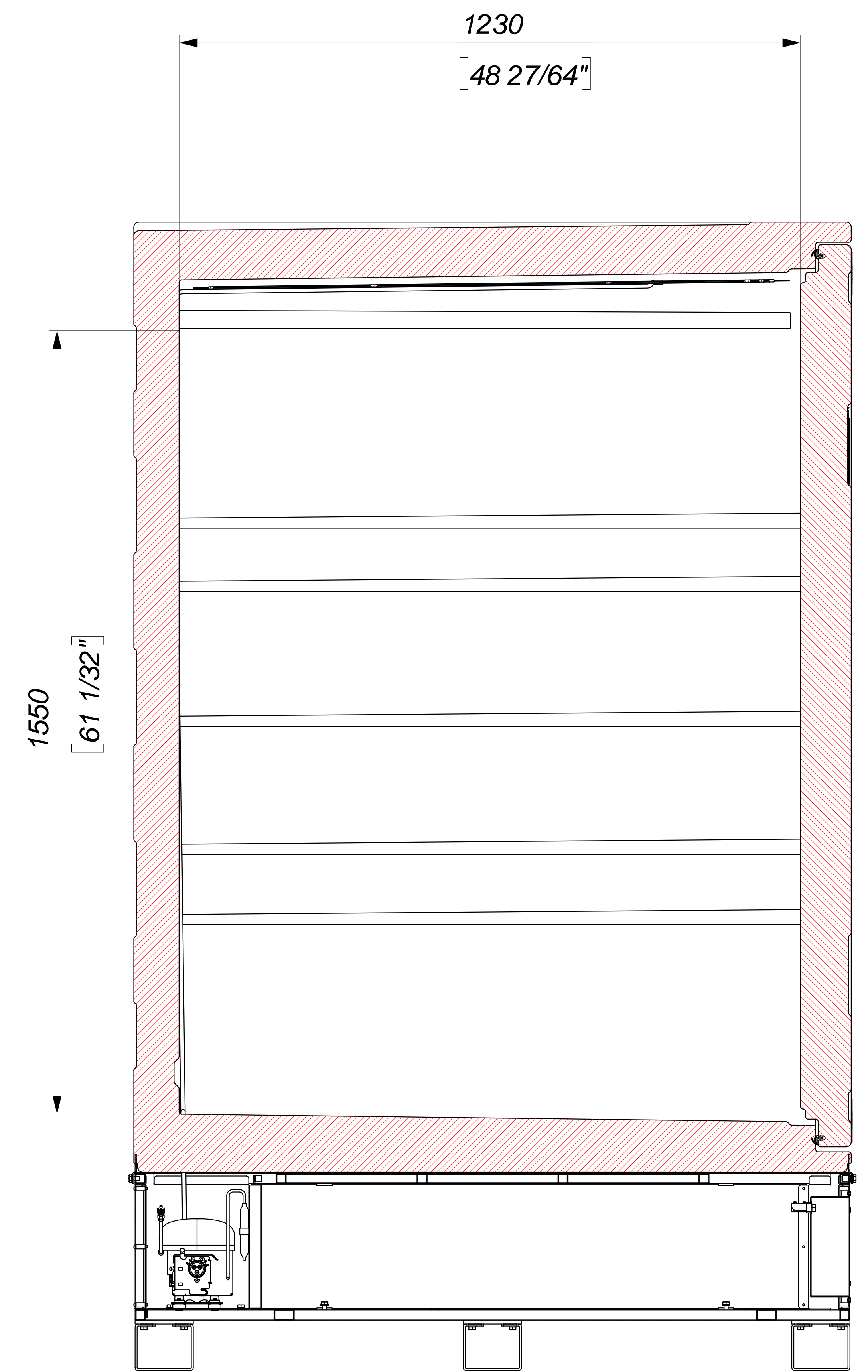
Sezione E-E SCALE 1 : 6
