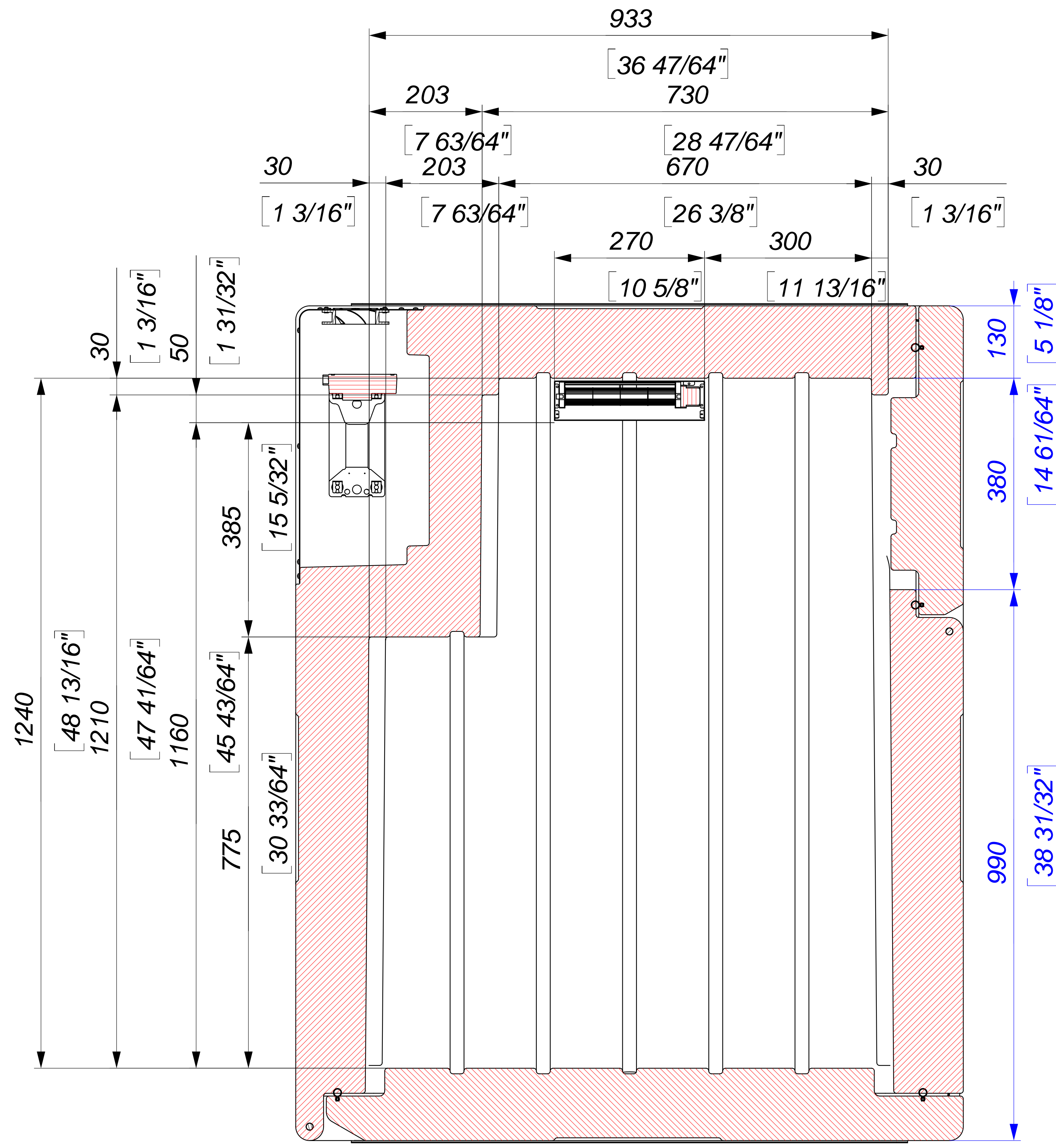
Sezione F-F SCALE 1:5
